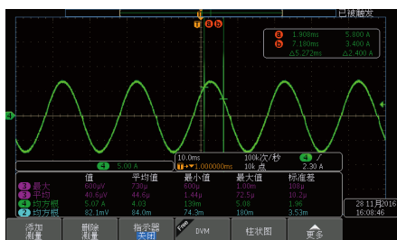
IT7600 三台并机实测均流
